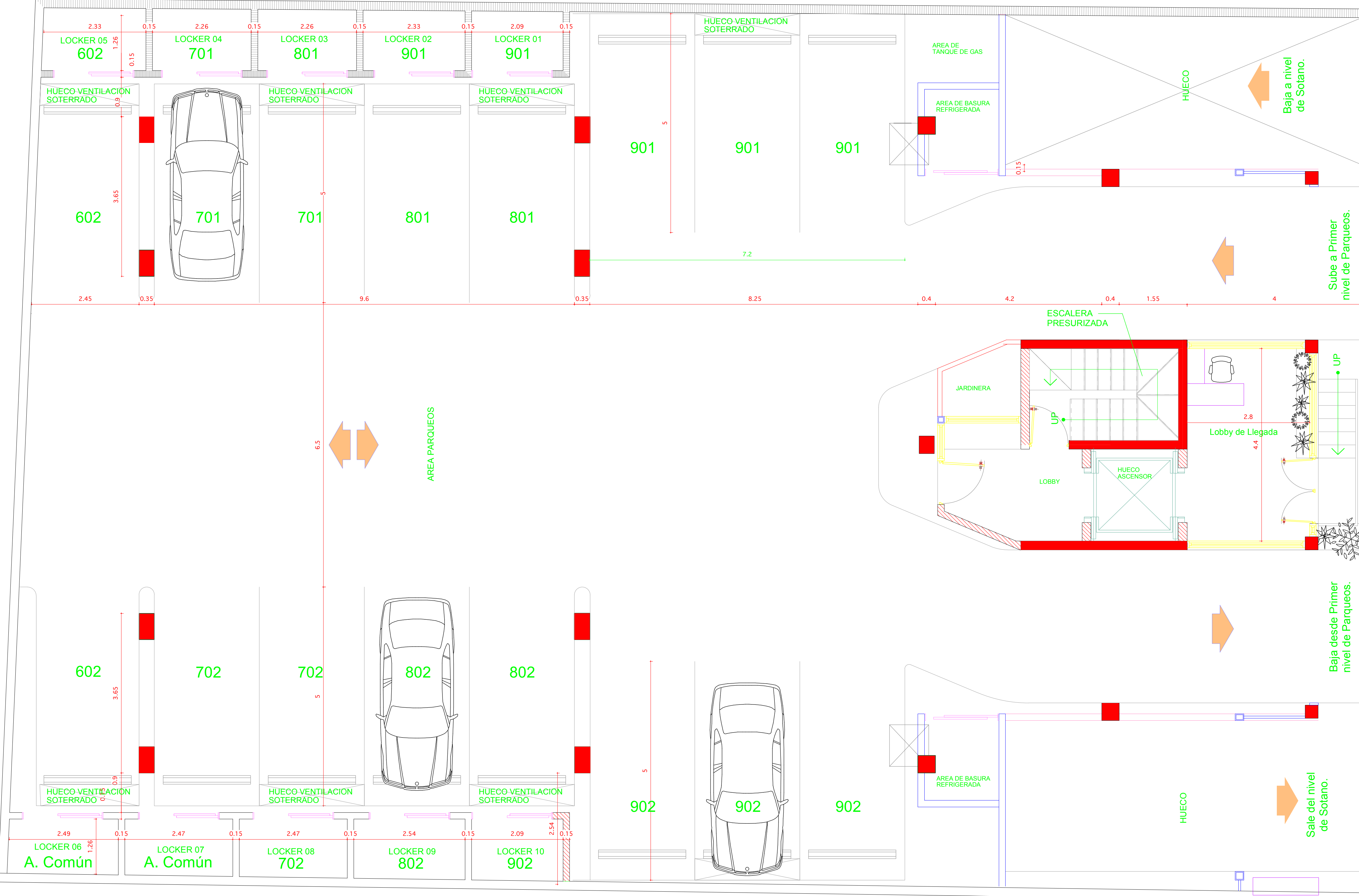
PLANTA DIMENSIONADA PARQUEOS 1er NIVEL
