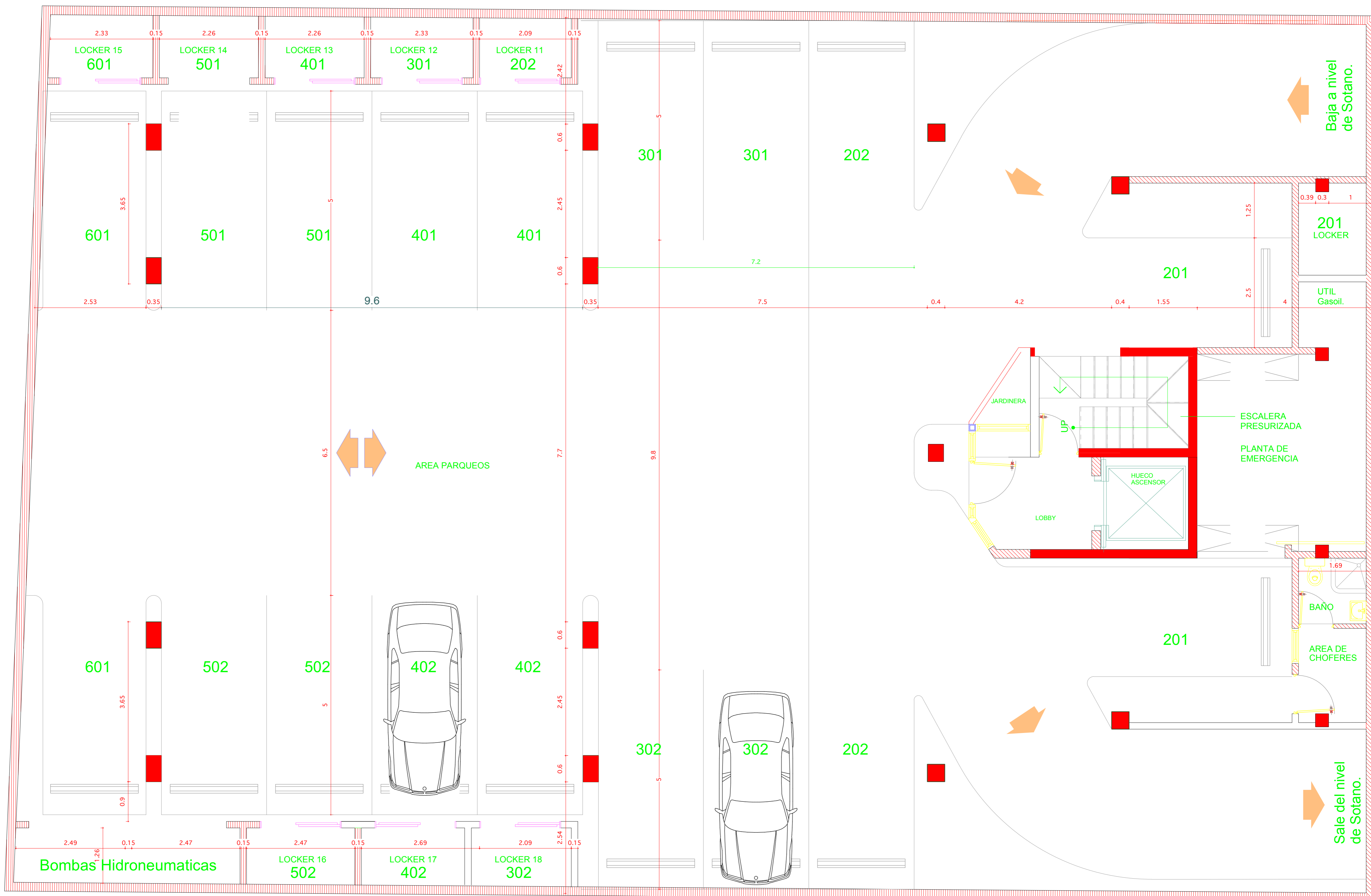
PLANTA DIMENSIONADA PARQUEOS NIVEL SOTERRADO
